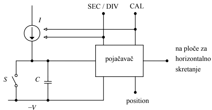
Slika 12. Sistem za horizontalno skretanje mlaza.
