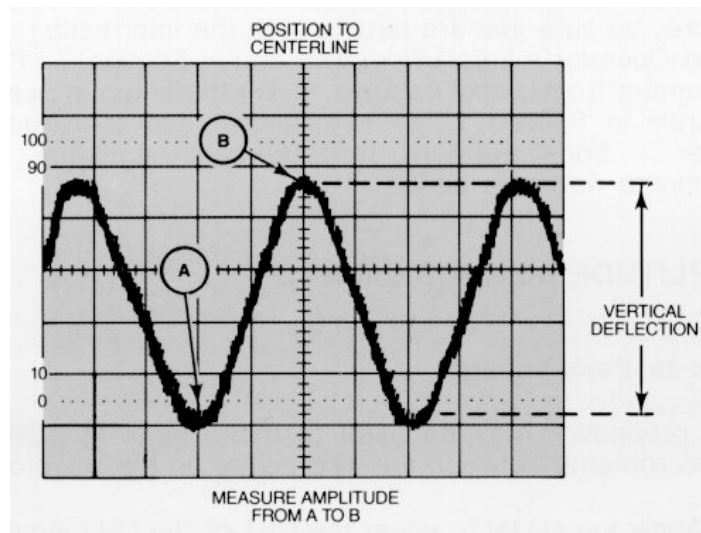
Slika 23. Merenje amplitude.
