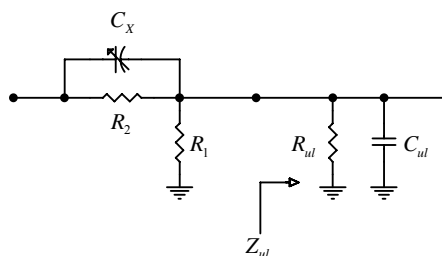
Slika 19. Sonda i ulazna impedansa osciloskopa.
